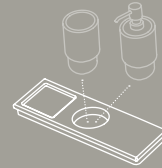
PORTA SAPONE CON FORO PER BICCHIERE O DISPENSER Soap holder with hole for glass or dispenser - ACMP3 30 x 12 x h2 pag. 810
