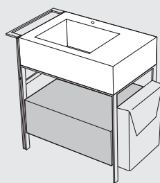
lavabo bacino sinistro con struttura, cassetto basso, portasciugamani e sacca (dx - sx)
