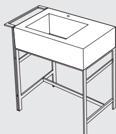
lavabo bacino sinistro con struttura e portasciugamani (dx - sx)
