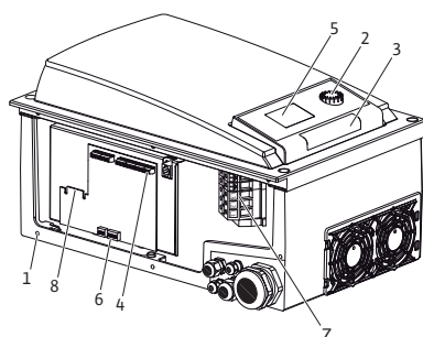
Fig. 9: Módulo electrónico
