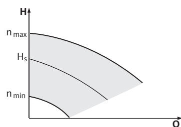
Fig. 44: Reguleringsdrift
