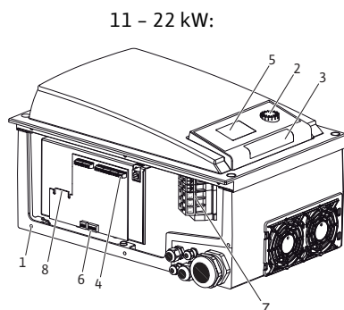
Fig. 9: Módulo electrónico
