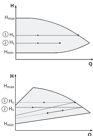
Fig. 43: Regolazione \Delta p\text{-}c/\Delta p\text{-}v
