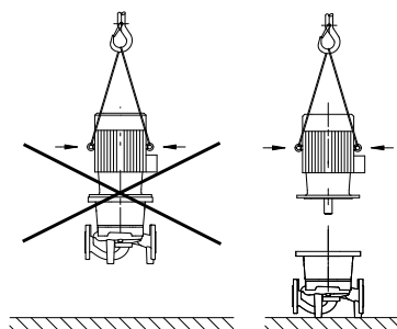
Fig. 8: Trasporto del motore
