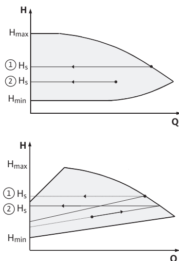
Fig. 43: Regulação \Delta p\text{-c}/\Delta p\text{-v}
