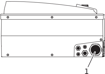
Fig. 23: Prensaestopas M25/M40
