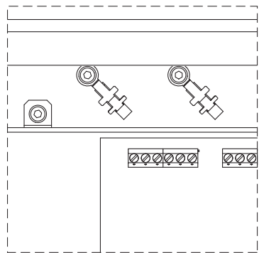
Fig. 24: Apantallamiento de los cables
