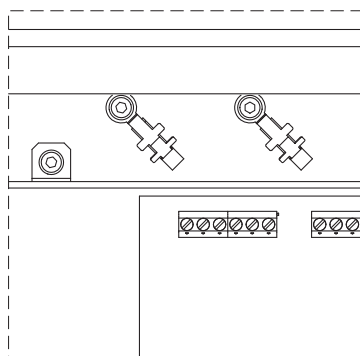
Fig. 24: Kabelafskærmning
