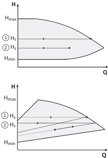
Fig. 43: Regulación \Delta p\text{-}c/\Delta p\text{-}v
