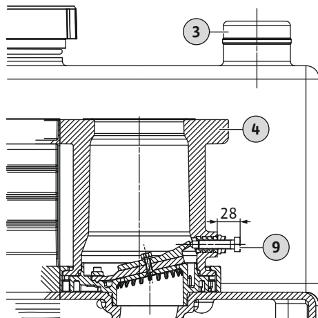
Fig. 8: Posizione della vite di aerazione
