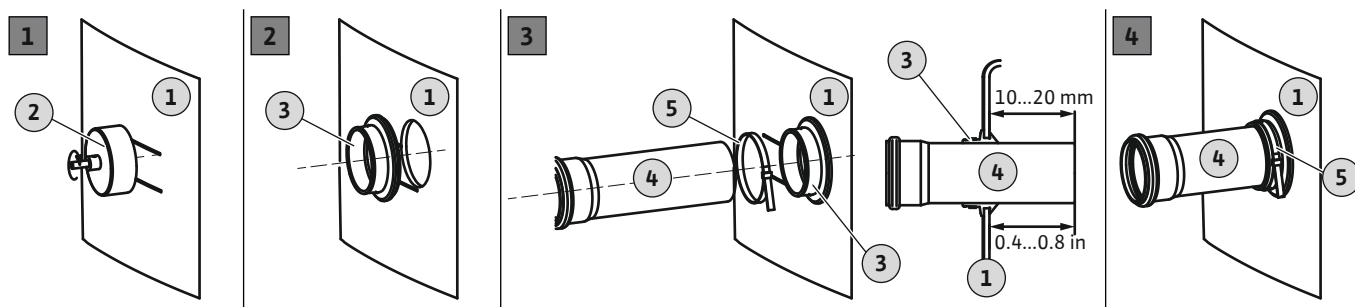
Fig. 5: Allacciamento dell'alimentazione
