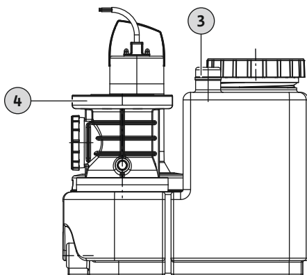
Fig. 6: Attacco ventilazione e disaerazione serbatoio di raccolta
