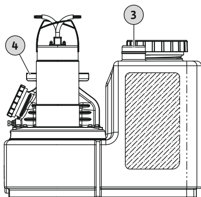
Fig. 6: Attacco ventilazione e disaerazione serbatoio di raccolta
