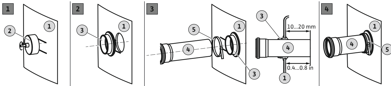
Fig. 5: Allacciamento dell'alimentazione
