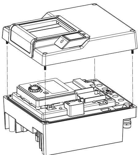
Fig. 108: Abrir a tampa do módulo eletrónico
