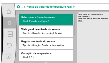
Fig. 62: Fonte do valor da temperatura real T1
