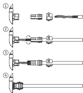
Fig. 24: Blindagem
