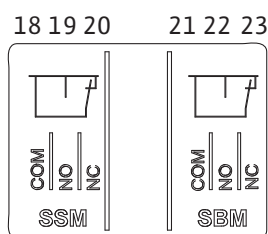
Fig. 23: Bornes para SSM y SBM
