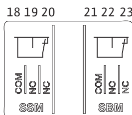
Fig. 23: Morsetti per SSM e SBM
