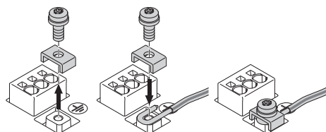
Fig. 22: Cable de conexión rígido
