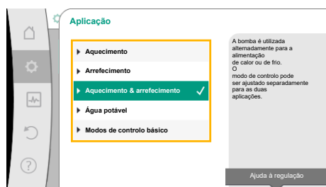
Fig. 45: Seleção da aplicação «Aquecimento & arrefecimento»
