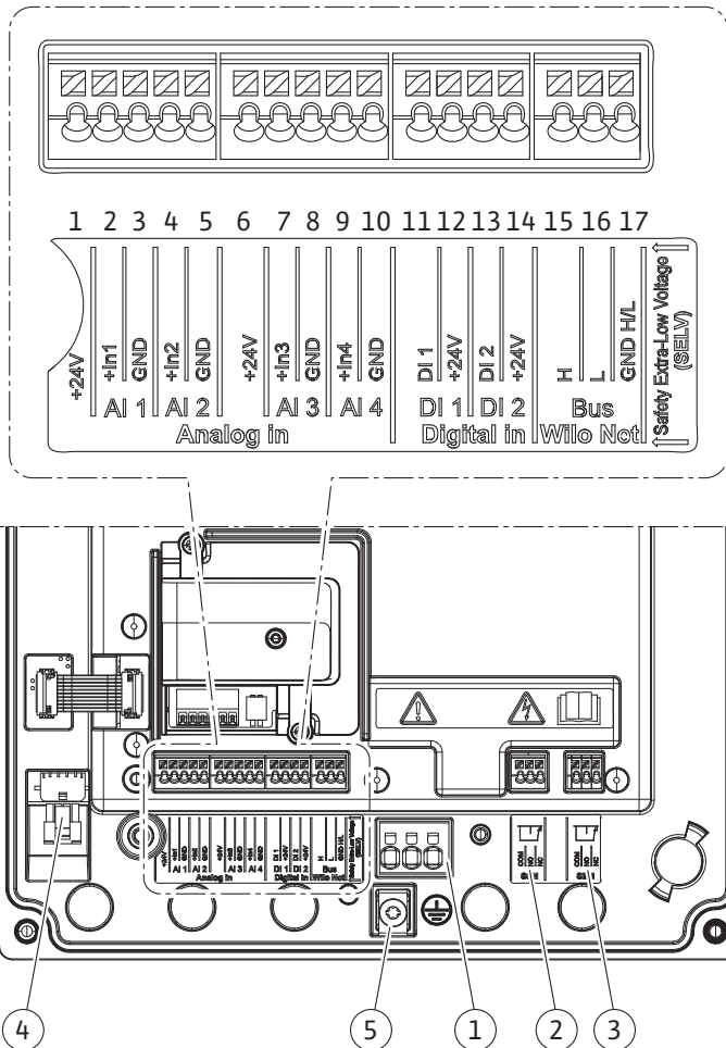
Fig. 19: Przegląd zacisków modułu
