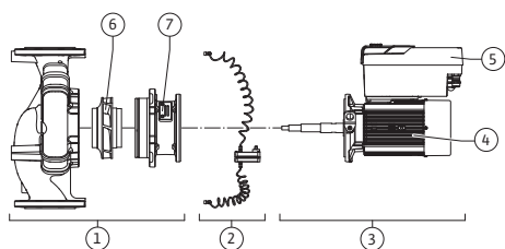
Fig. 3: Podzespoły funkcjonalne
