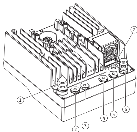
Fig. 18: Pressacavi/passacavi
