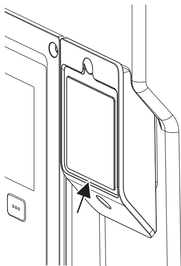
Fig. 27: Tampa para o módulo Wilo-Smart Connect BT
