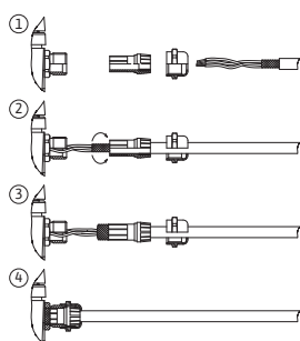
Fig. 24: Supporto schermato
