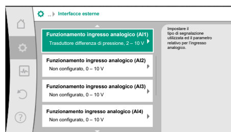
Fig. 67: Funzione ingresso analogico
