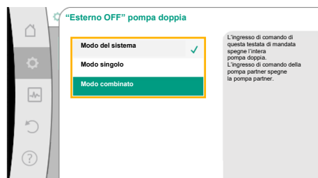
Fig. 65: Modalità selezionabili per EXT. OFF delle pompe doppie
