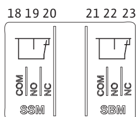
Fig. 23: Zaciski SSM i SBM
