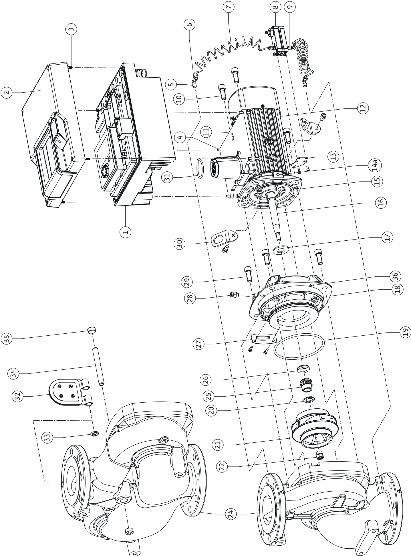
Fig. I: Stratos GIGA2.0-I /Stratos GIGA2.0-D – DN 100; 1,1 ... 1,5 kW
