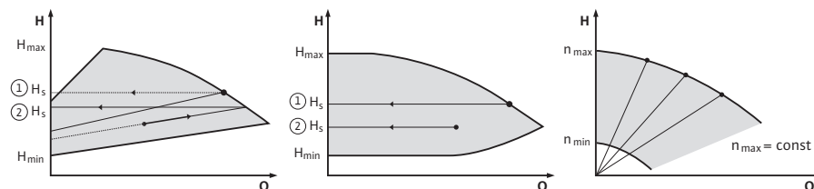
Fig. 37: Funciones de regulación
