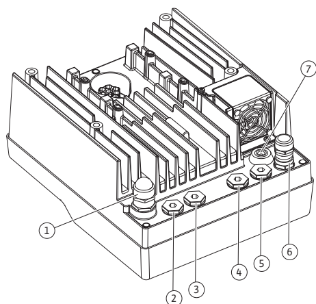
Fig. 19: Prensaestopas/pasamuros
