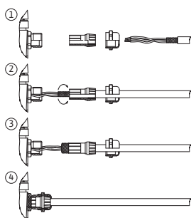
Fig. 25: Supporto schermato
