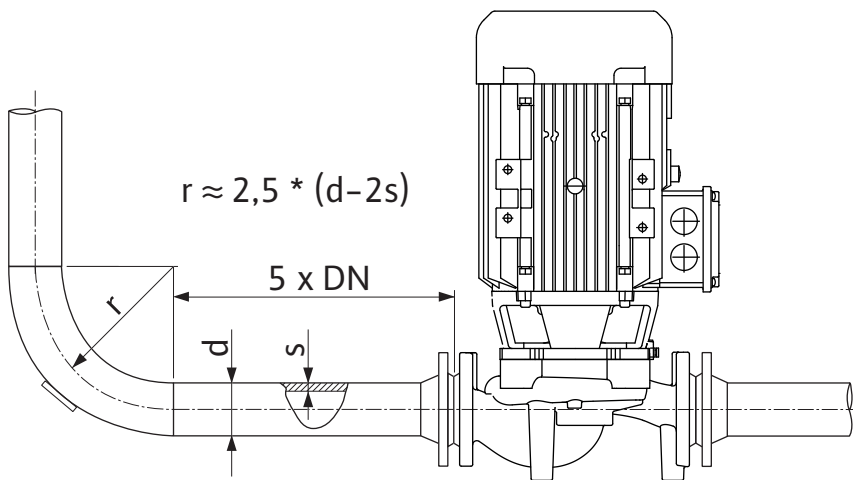
Fig. 12: Percurso de estabilização antes e depois da bomba
