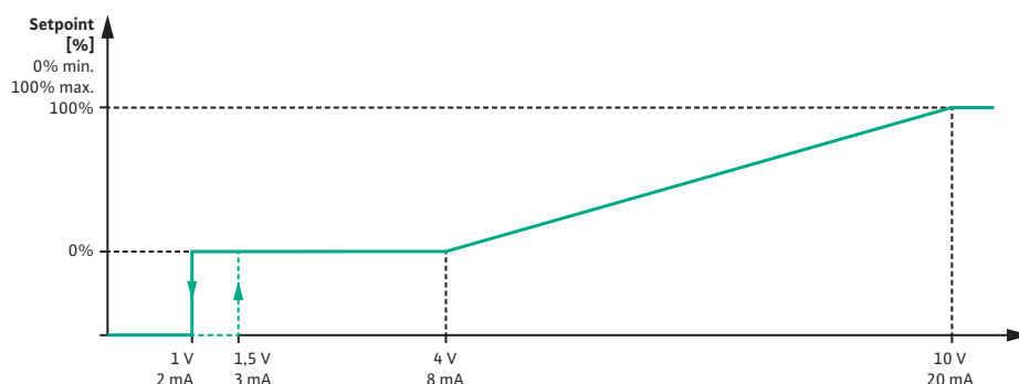
Fig. 79: Zachowanie wejścia analogowego AI2: Wartość zadana przy typie sygnału 0 ... 10 V / 0 ... 20 mA
