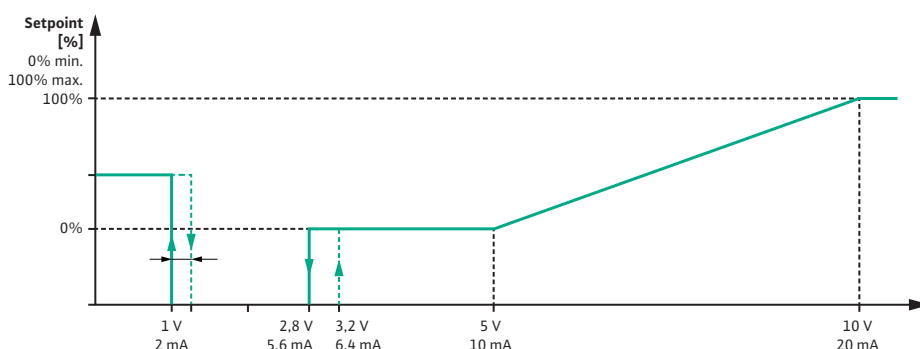
Fig. 78: Comportamiento de la entrada analógica AI2: Valor de consigna para el tipo de señal 2 ... 10 V / 4 ... 20 mA
