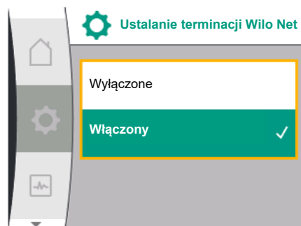
Fig. 81: Menu Ustawianie terminu Wilo Net
