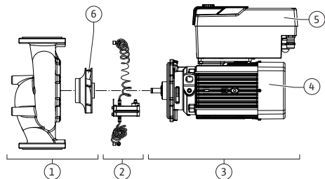
Fig. 3: Moduli funzionali
