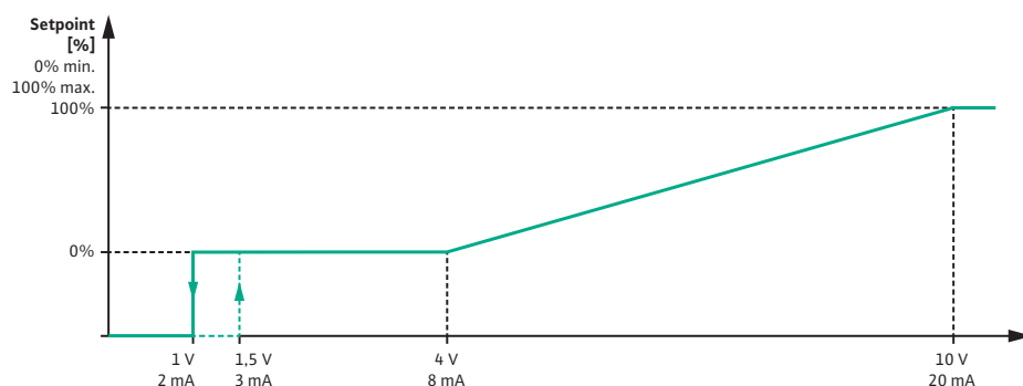
Fig. 79: Comportamento segnale analogico AI2: Valore di consegna per tipo di segnale 0 ... 10 V / 0 ... 20 mA
