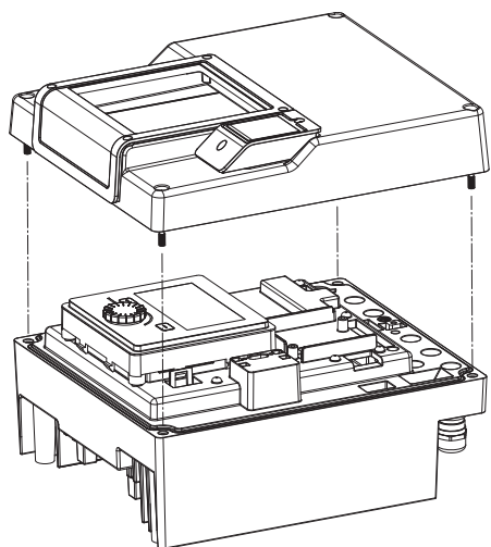
Fig. 105: Abrir a tampa do módulo eletrónico
