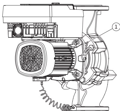
Fig. 11: Wypchnięcie głowicy silnika przez gwintowane otwory (DN 100 ... DN 125)
